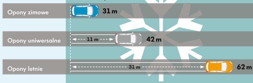
Hamowanie na śniegu: wyniki dla prędkości 50 km/h na ośnieżonej drodze
