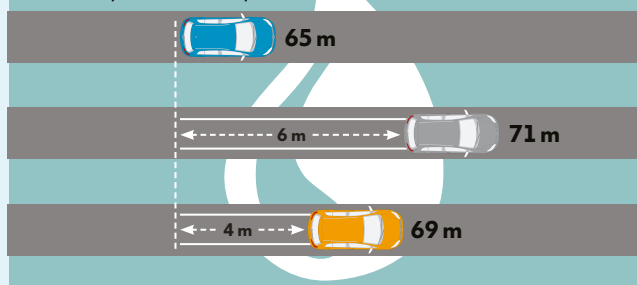
Hamowanie w deszczu: wyniki dla prędkości 100 km/h na mokrej drodze w temperaturze około 5°C
